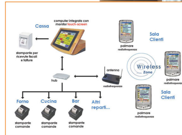
L'INGEGNER GOTTARDI, TITOLARE DI VERONA SOFTWARE, ILLUSTRA LE CARATTERISTICHE DEL SISTEMA COMPUTERIZZATO PER LA GESTIONE DELLE COMANDE. A LATO, LO SCHEMA DELL'IMPIANTO.
